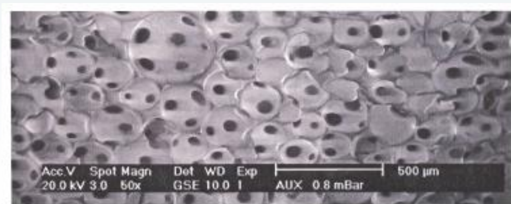
Микрофотография, показывающая структуру пенополиуретана.
